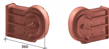
About de rive universelle gauche à recouvrement Réf. 1072
