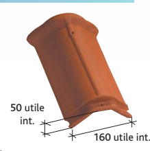
Faîtière / arêtier grand modèle à emboîtement (3 au ml) Réf. 706 Crochet adapté : crochet F6-Réf. CRP 706/706
