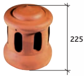
Lanterne grand modèle Ø 120 utile (Section aération 80 cm²) Réf. 1001
