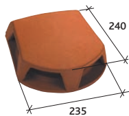
Lanterne bi-section Ø 120 utile et Ø 150 utile (Section aération : 130 cm²) Réf. 1000
