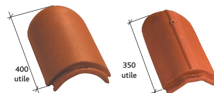
About d'arêtier 1/2 rond (1) à emboîtement grand modèle Réf. 851
