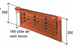
Rive individuelle droite à recouvrement Delta 10 (2,6 au ml au pureau de 390 mm) Réf. 202.41
